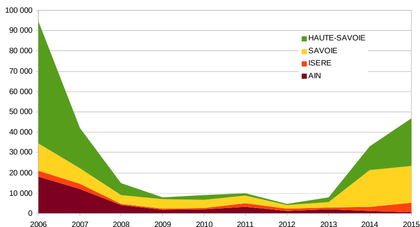
Volumes de bois scolytés en forêts relevant du régime forestier dans les Alpes du Nord Evolution 2006 - 2015
